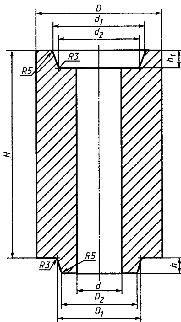
Рисунок 1 - Стопорная трубка номеров 1-8 и 8-1
