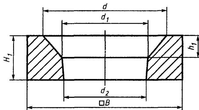
Рисунок 10 - Верхняя часть составного гнездового кирпича номер 45
