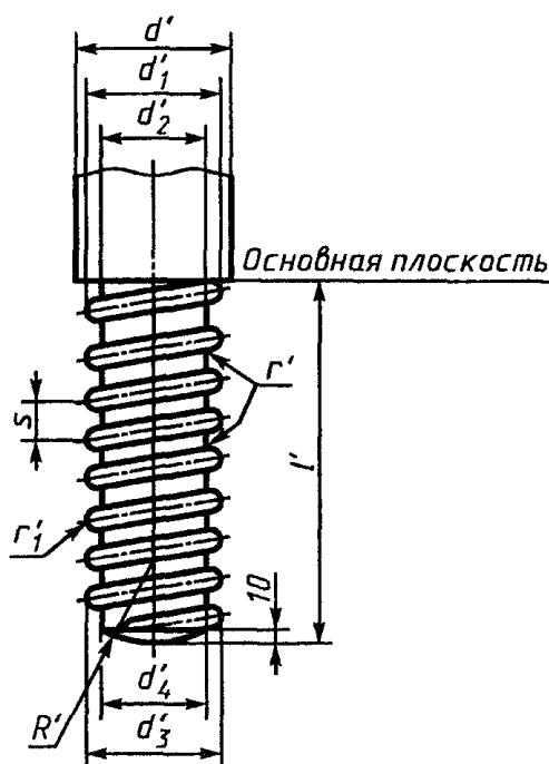
Рисунок Б.1- Винтовая нарезка металлического стопорного штыря
