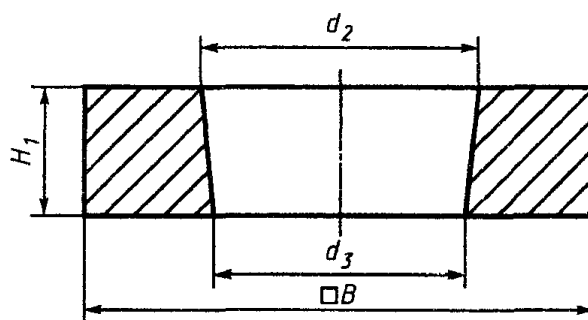
Рисунок 11 - Нижняя часть составного гнездового кирпича номер 46
