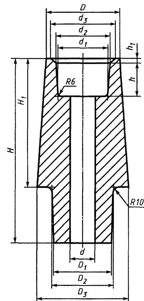
Рисунок 7 - Стакан номеров 33 и 34
