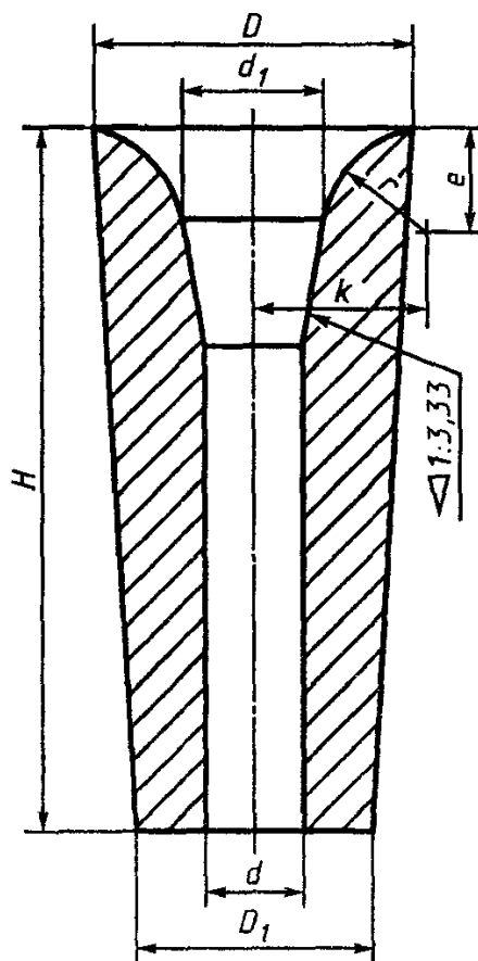
Рисунок 3 - Стакан номеров 15 - 23
