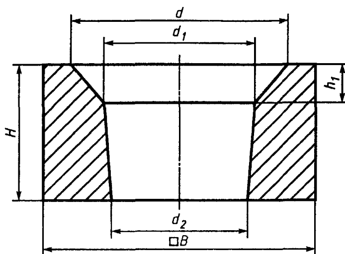
Рисунок 9 - Гнездовой кирпич номеров 37 - 44
