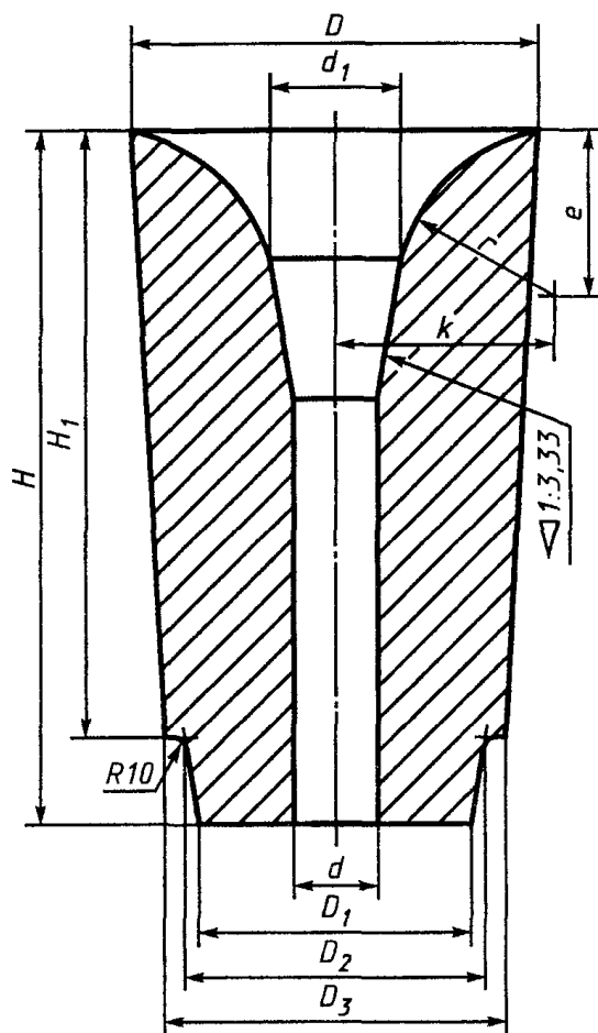
Рисунок 4 - Стакан номер 24
