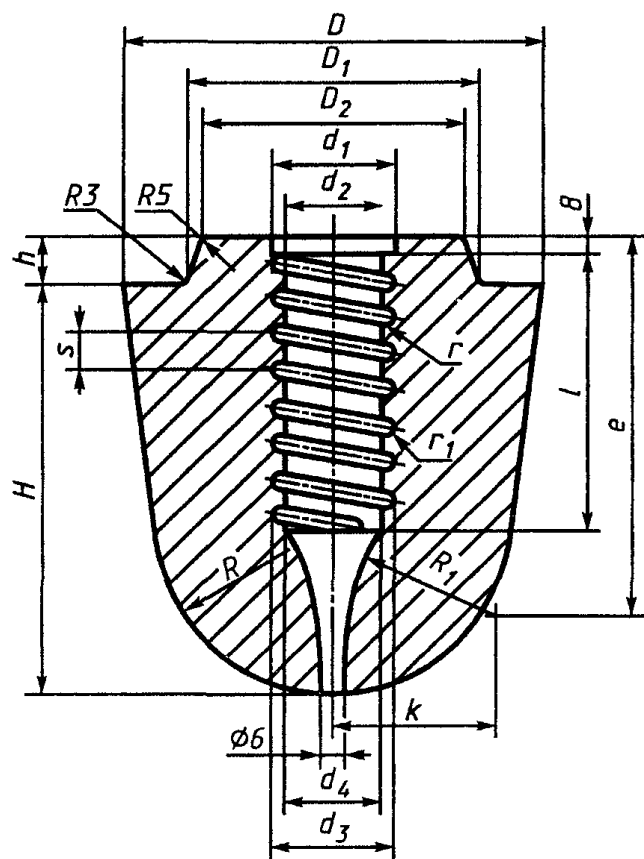
Рисунок 2 - Пробка номеров 9 - 14, 14-1, 14-2
