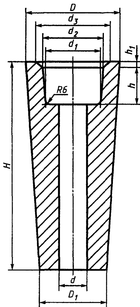
Рисунок 5 - Стакан номеров 25 - 30
