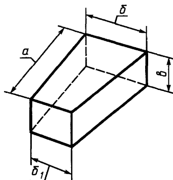
Рисунок 3 — Трапецеидальный кирпич
