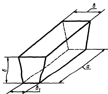
Рисунок 2 — Ребровый клин
